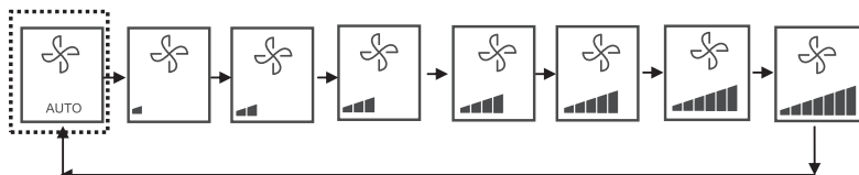
Рис. 28. Последовательность переключения 7 скоростей вращения вентилятора.
