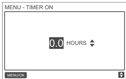
Рис. 42. Настройка TIMER ON [Включение по таймеру]
