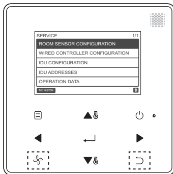
Рис. 15 - Доступ к меню настройки параметров
