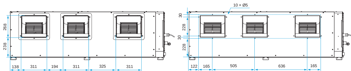
Размеры монтажного отверстия воздуховода после снятия фланца для подачи воздуха
